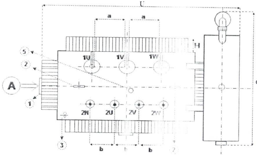
ÜSTTEN GÖRÜNÜM
