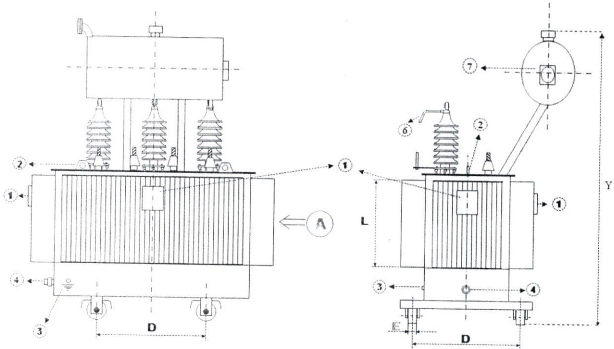
ÖNDEN GÖRÜNÜM
