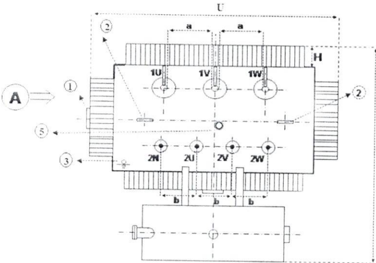
ÜSTTEN GÖRÜNÜM
