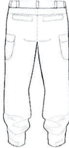
ARKADAN GÖRÜNÜM
