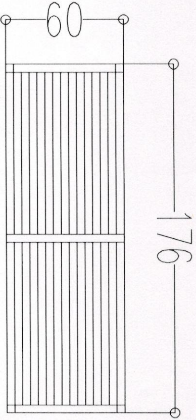
BANK 1 PLAN 60X60X176 YÜZEY KUTU PROFİLLER 4 CM ARAYLA ATILACAKTIR
